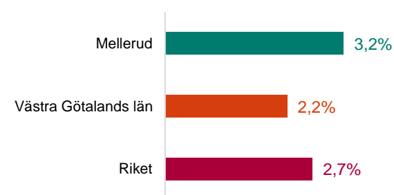
Figur 26: Långtidsarbetslöshet
