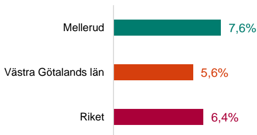
Figur 26: Långtidsarbetslöshet
